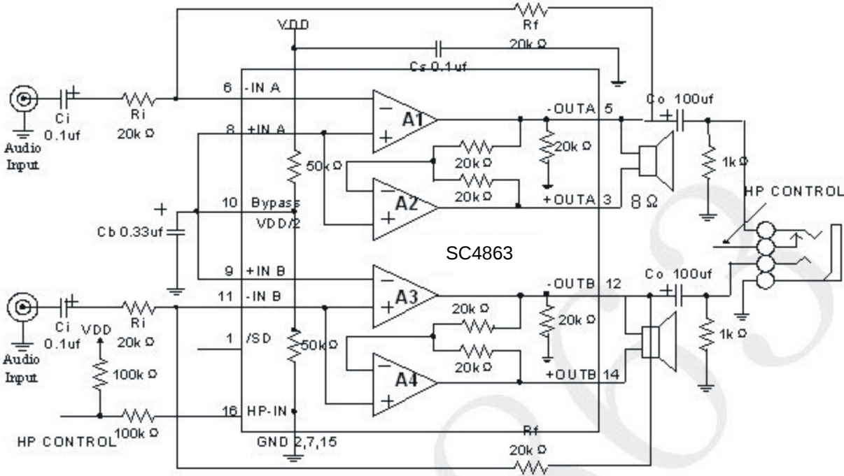
SC4863应用电路图
