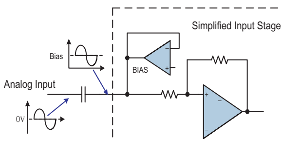
图4 模拟输入级等效模型
