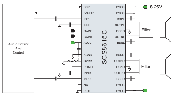
图6 SCS8615C单端输入接法
