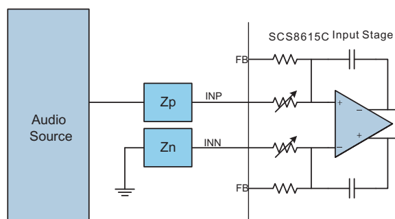
图7 匹配输入阻抗
